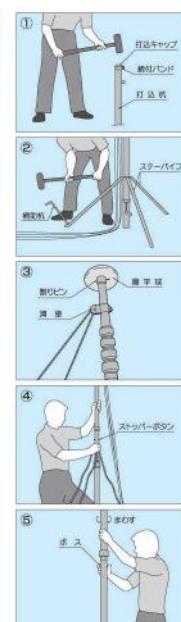
スカイボール (埋込自立式伸縮ポール、アルミ合金製)
